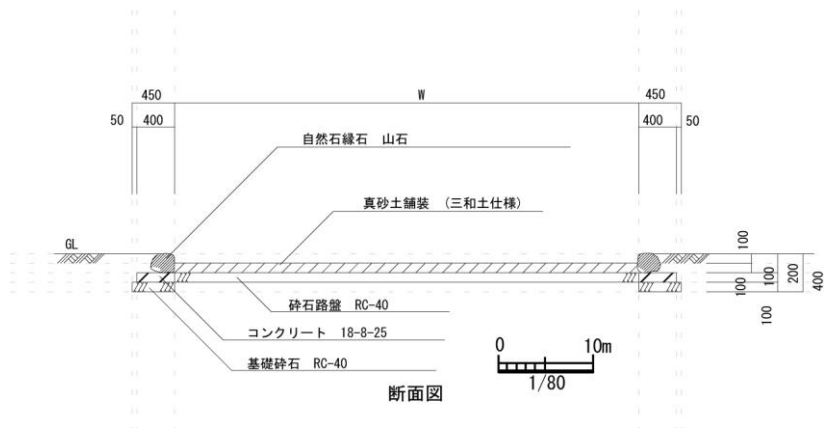
図 4-21 南堀跡表示標準断面図
