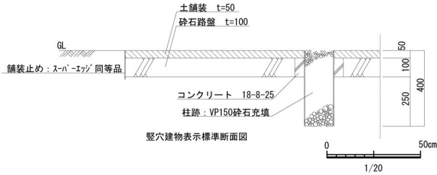
図 4-27 竪穴建物跡表示詳細図
