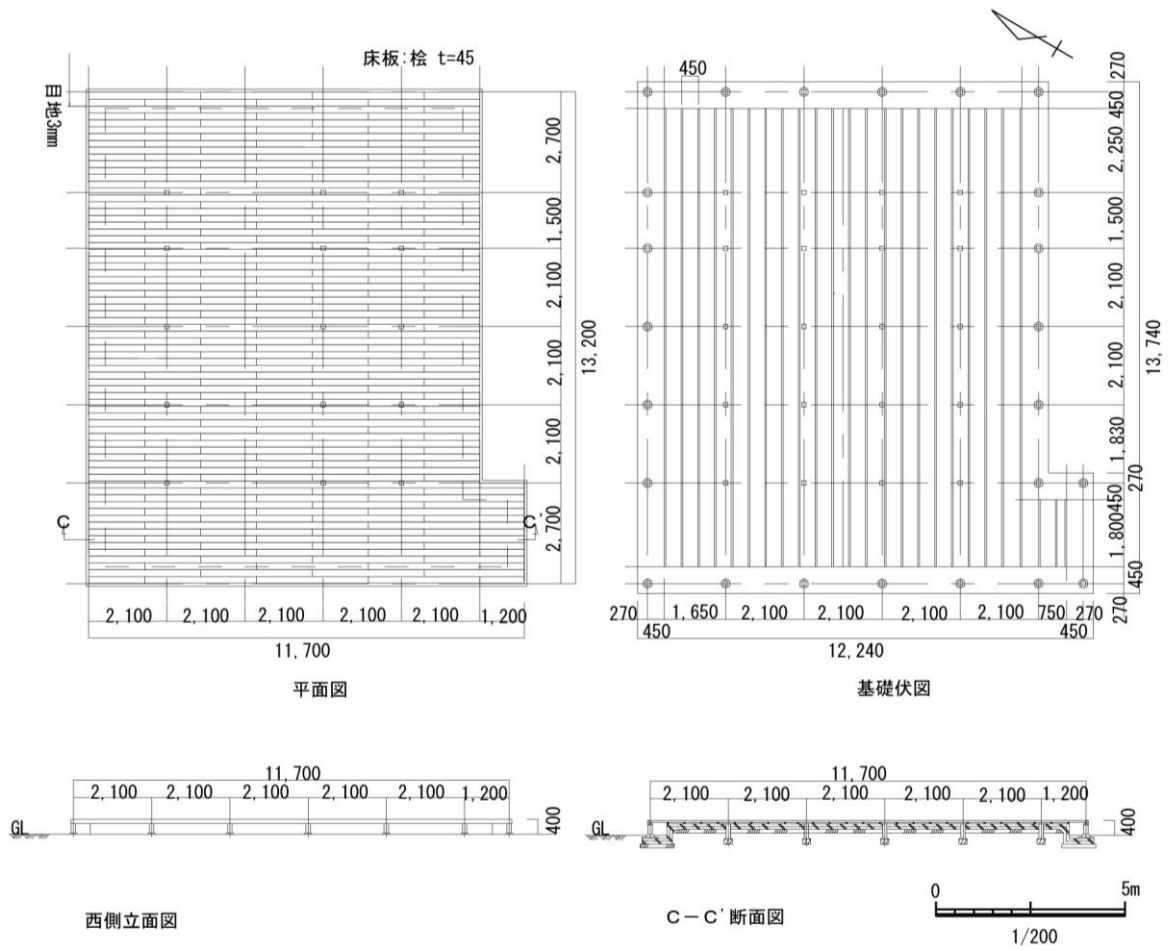
図 4-15 礎石建物跡 SB42 表示詳細図
