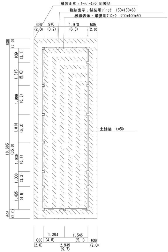
SB05掘立柱建物表示平面図
