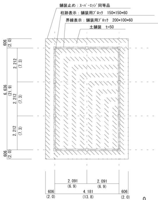
SB11掘立柱建物表示平面図
