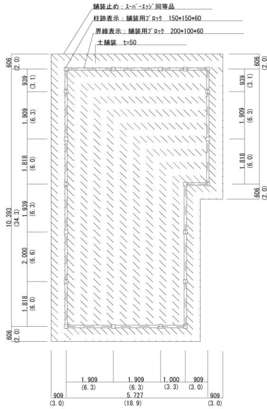
SB02掘立柱建物表示平面図
