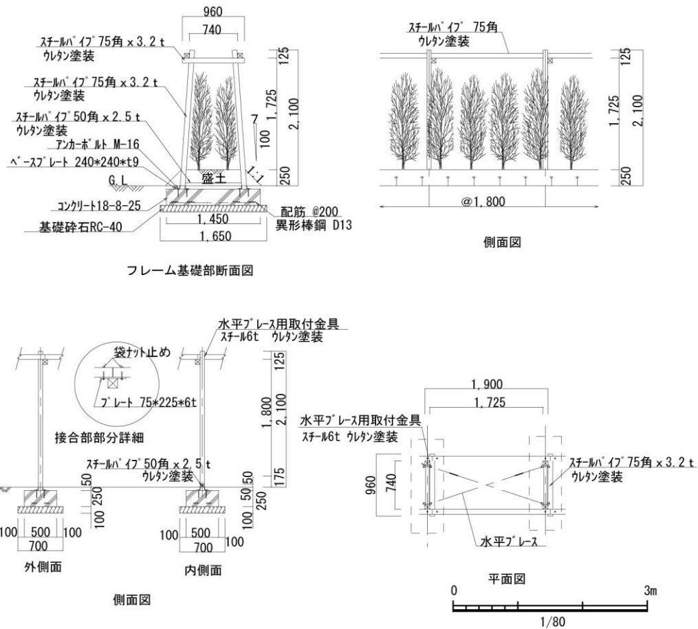
図 4-18 土塀跡表示詳細図
