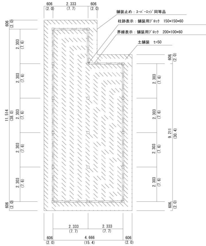
SB23掘立柱建物表示平面図
