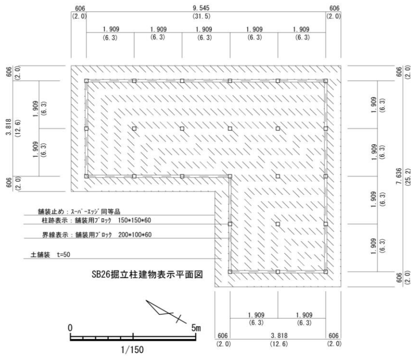
図 4-24 掘立柱建物跡 (SB23・SB26) 表示平面図
