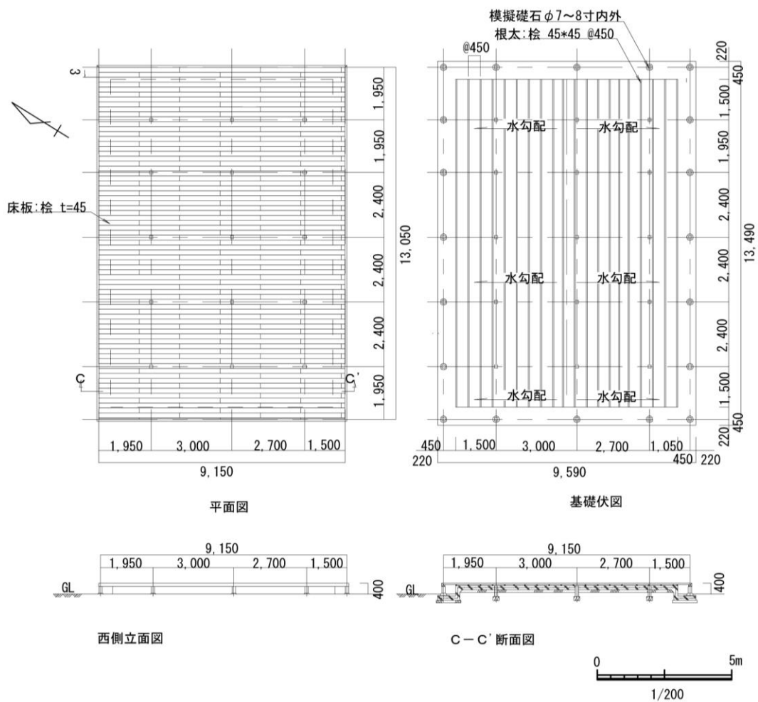
図 4-14 礎石建物跡 SB41 表示詳細図
