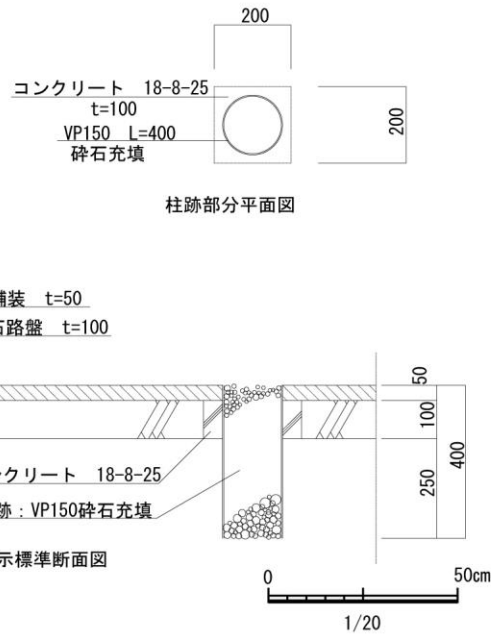
図 4-27 竪穴建物跡表示詳細図
