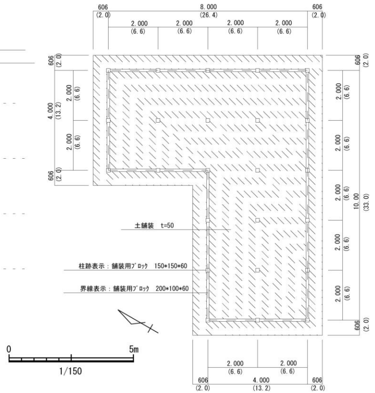
SB17掘立柱建物表示平面図
