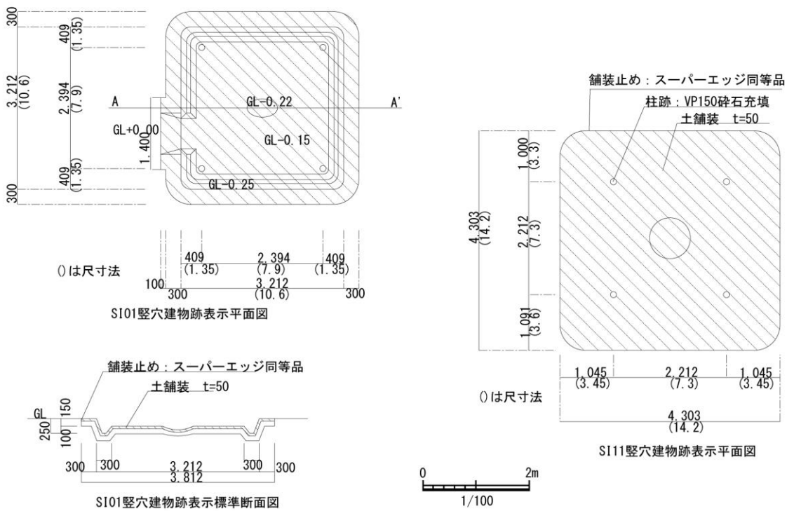
図 4-28 竪穴建物跡 (SI01・SI11) 表示平面図
