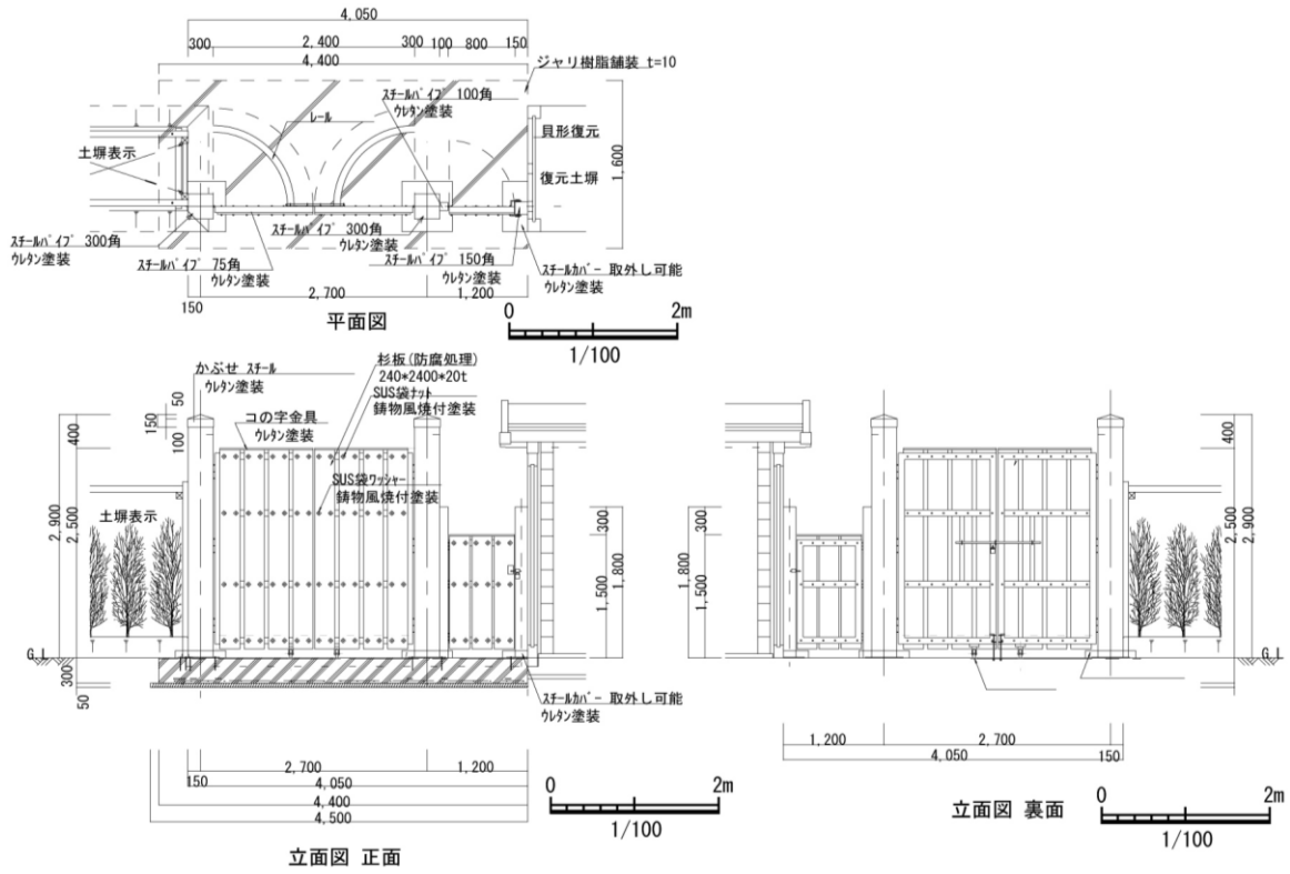
図 4-19 協門跡表示詳細図
