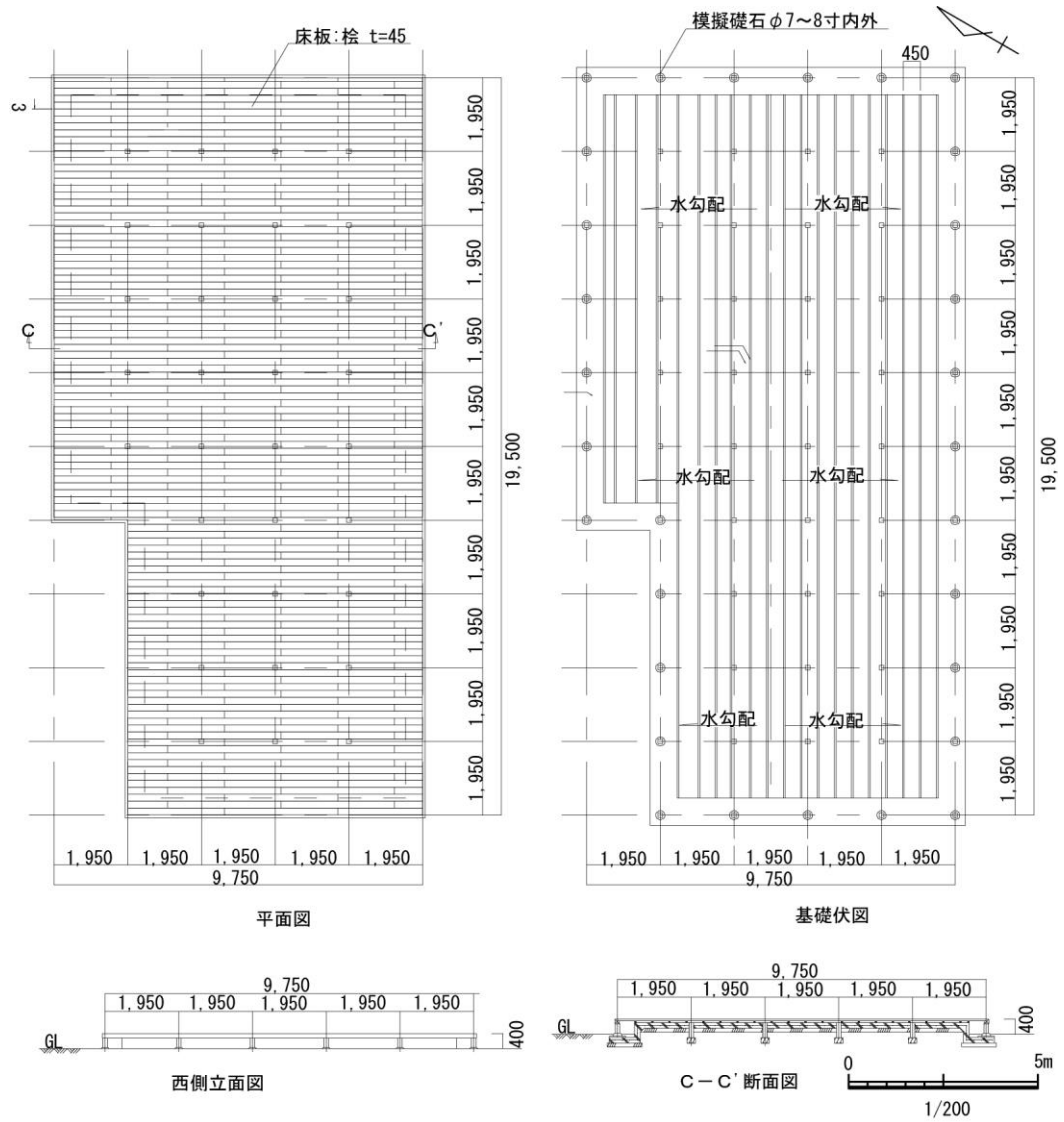
図 4-16 礎石建物跡 SB44 表示詳細図
