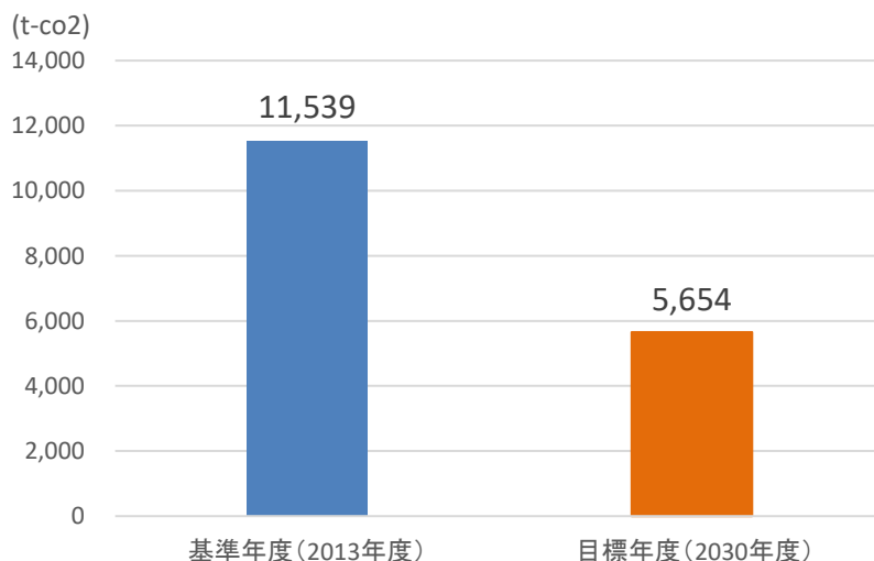
温室効果ガスの削減目標
