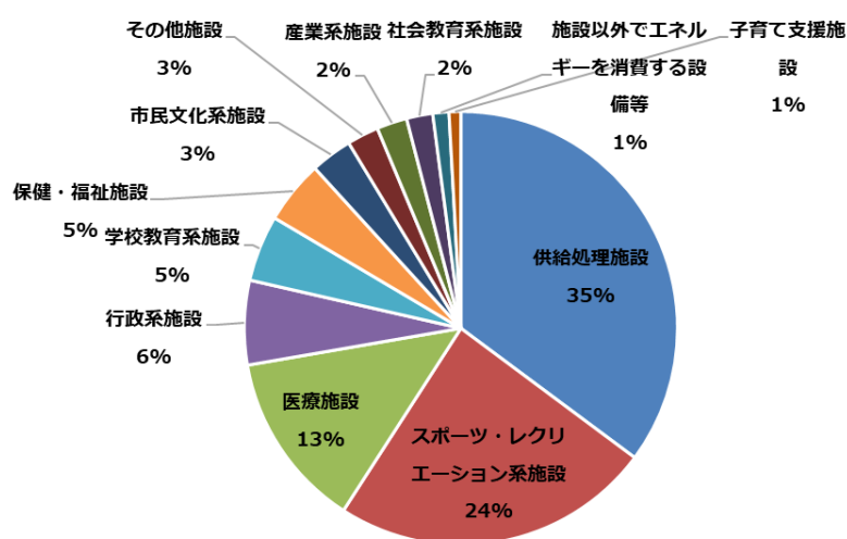
施設別の「温室効果ガス総排出量」の割合（2022 年度）
