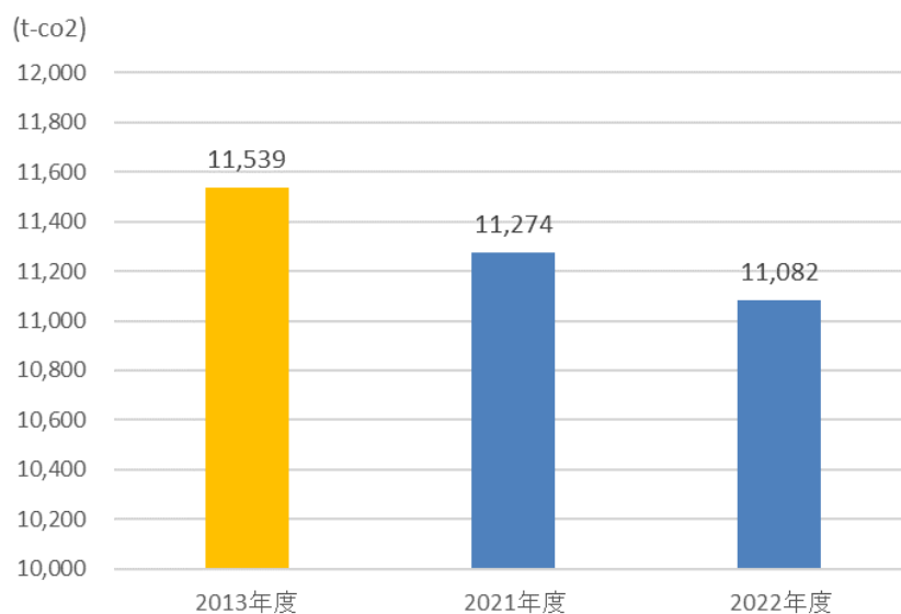
飛騨市の事務・事業に伴う「温室効果ガス総排出量」の推移
