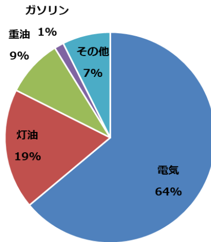
エネルギー種別の「温室効果ガス総排出量」の割合（2022 年度）
